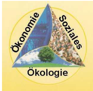
drei-Seiten eines Dreiecks
